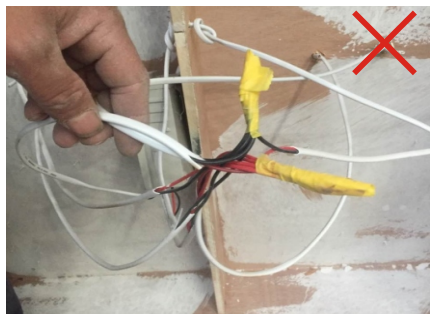
接线不得仅用胶布缠绕
