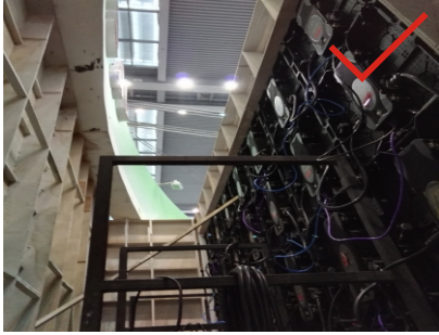
操作间封顶, 不合格 操作间未封顶, 合格 带有电视墙或其他电路设备的操作间必须散热良好, 不得封顶。
