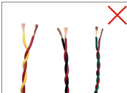
各类麻花线、双绞线：禁用
