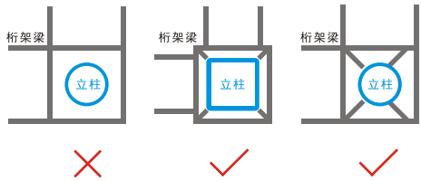
桁架升降支撑结构截面示意图
